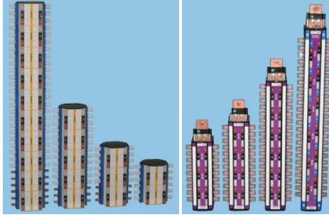
انظمة توزيع نحاس 100 الى 800 امبير
